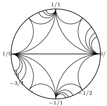
图 2: Farey 图的圆盘模型
